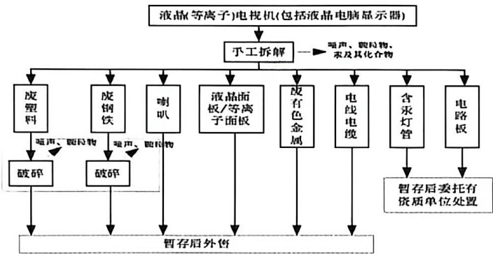
图 2-3 液晶电视机/液晶显示器拆解工艺流程及产污节点图
